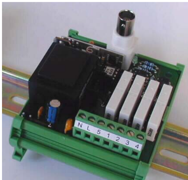
Funkfernsteuer-Empfänger EFB-EK4-UM72-BNC
